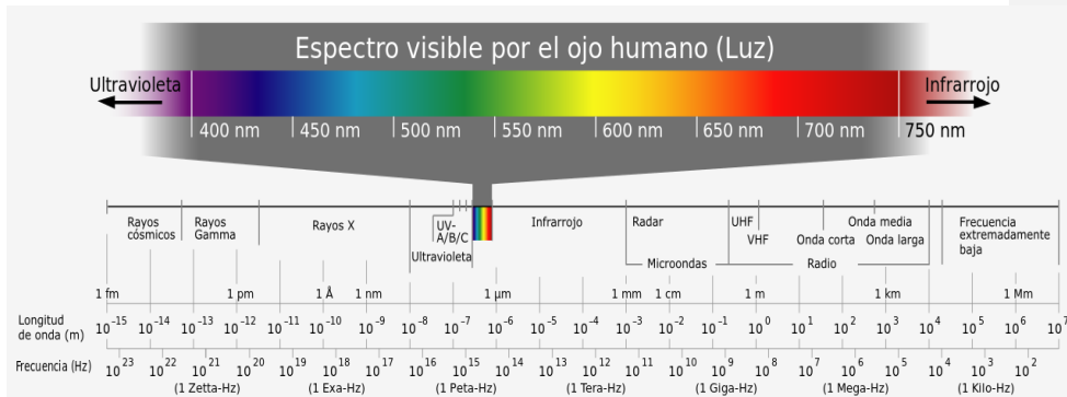
Fig. 1: Espectro electromagnético
