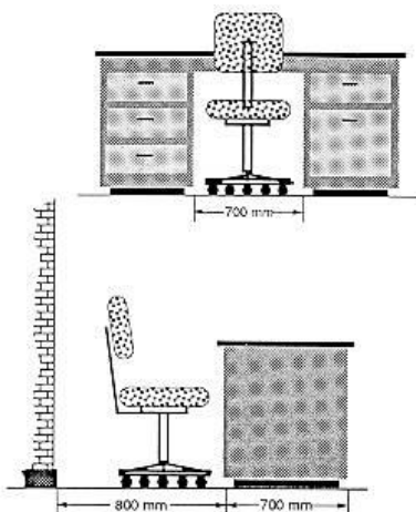
Figura 2: cotas de emplazamiento para las piernas en puestos de trabajo sentados
