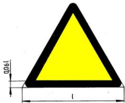
Señales de advertencia Figura 2
